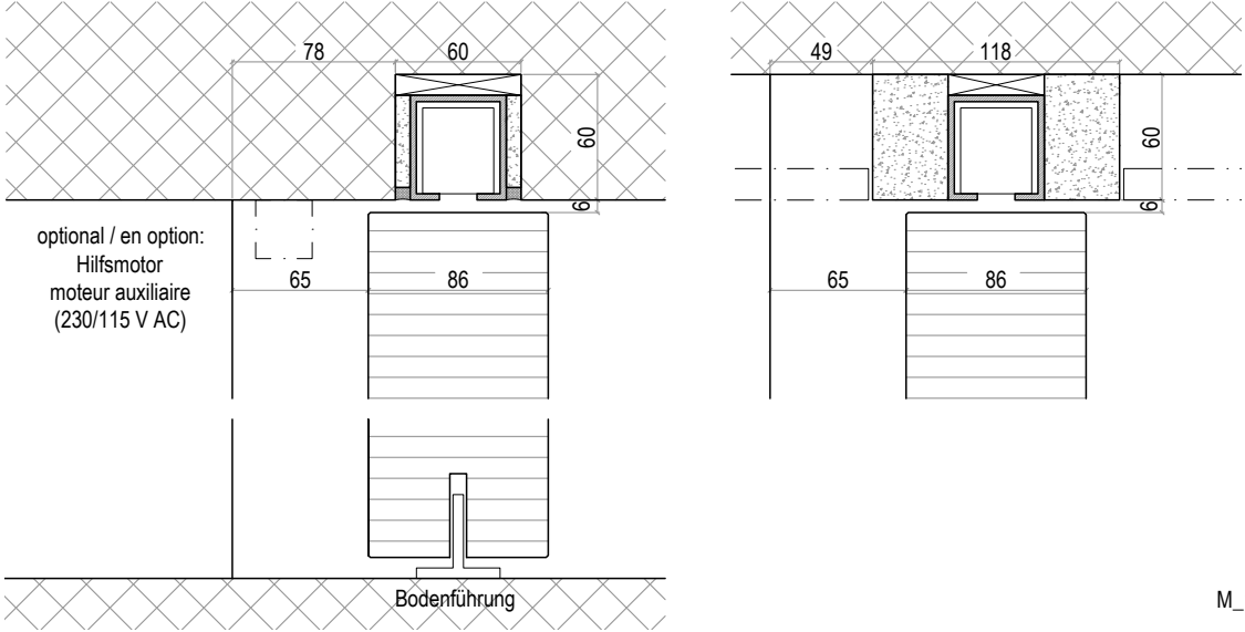
Sturzdetail/Bodendetail (Vertikalschnitt)
