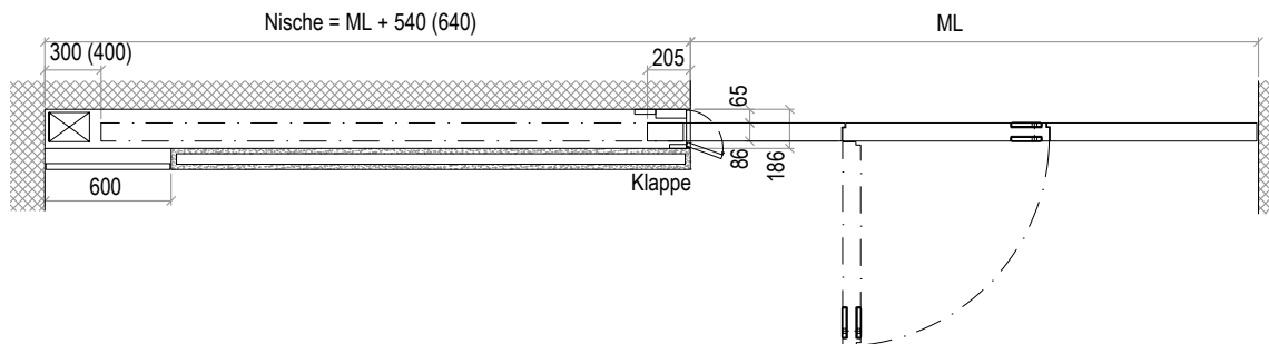
Ausführungsvariante mit Fluchttüre, Massangaben (Horizontalschnitt)
