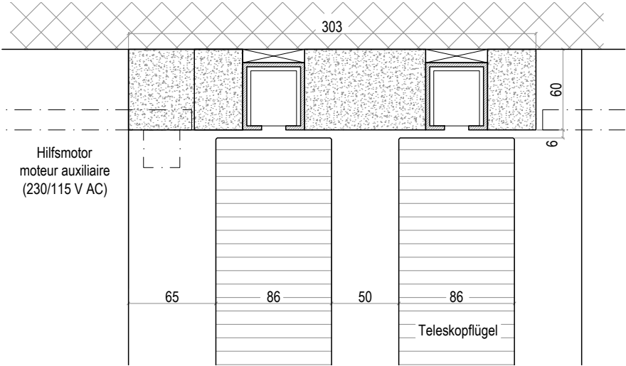
Ausführungsvariante (Vertikalschnitt)
