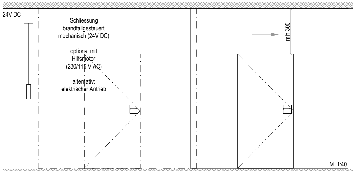
Ausführungsvariante mit Fluchttüre (Ansicht)
