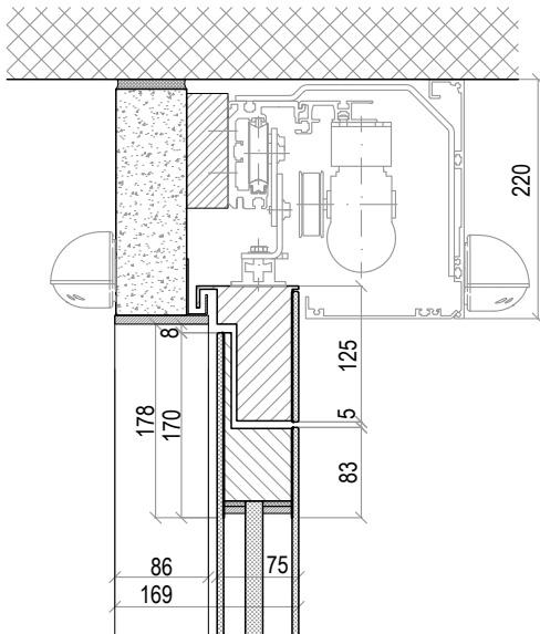
Ausführungsvarianten DELTAGLISS, Sturzdetail (Vertikalschnitt)
