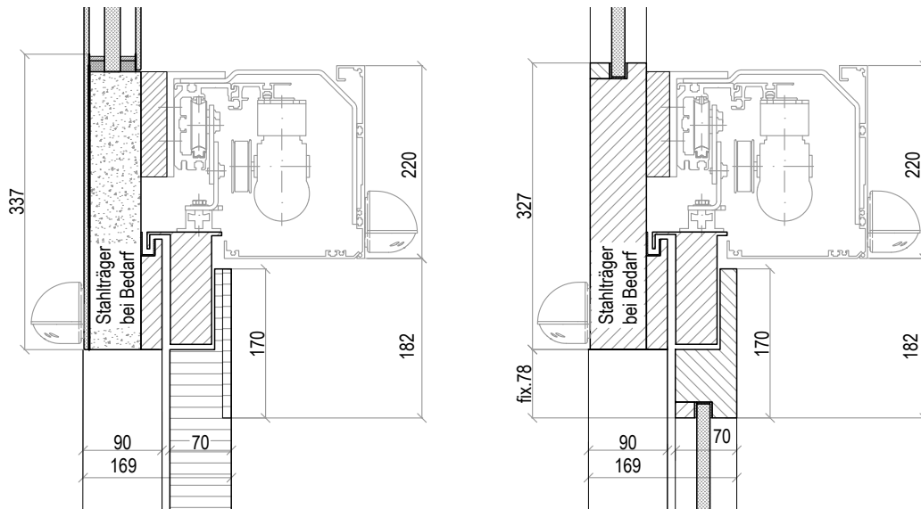
Ausführungsvarianten FIREGLISS und FRAMEGLISS, Sturzdetail (Vertikalschnitt)
