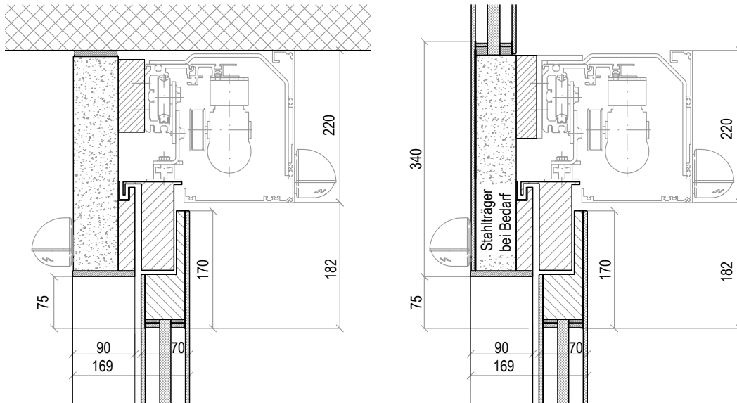
Ausführungsvarianten DELTAGLISS, Sturzdetail (Vertikalschnitt)
