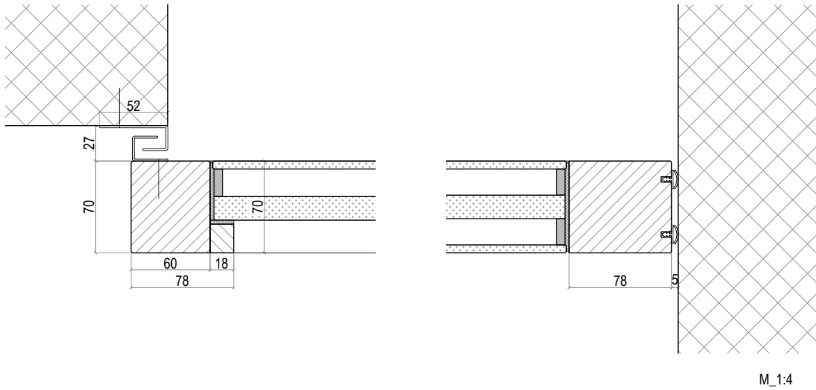
Varianten 1-flüglige Ausführung (Horizontalschnitt)
