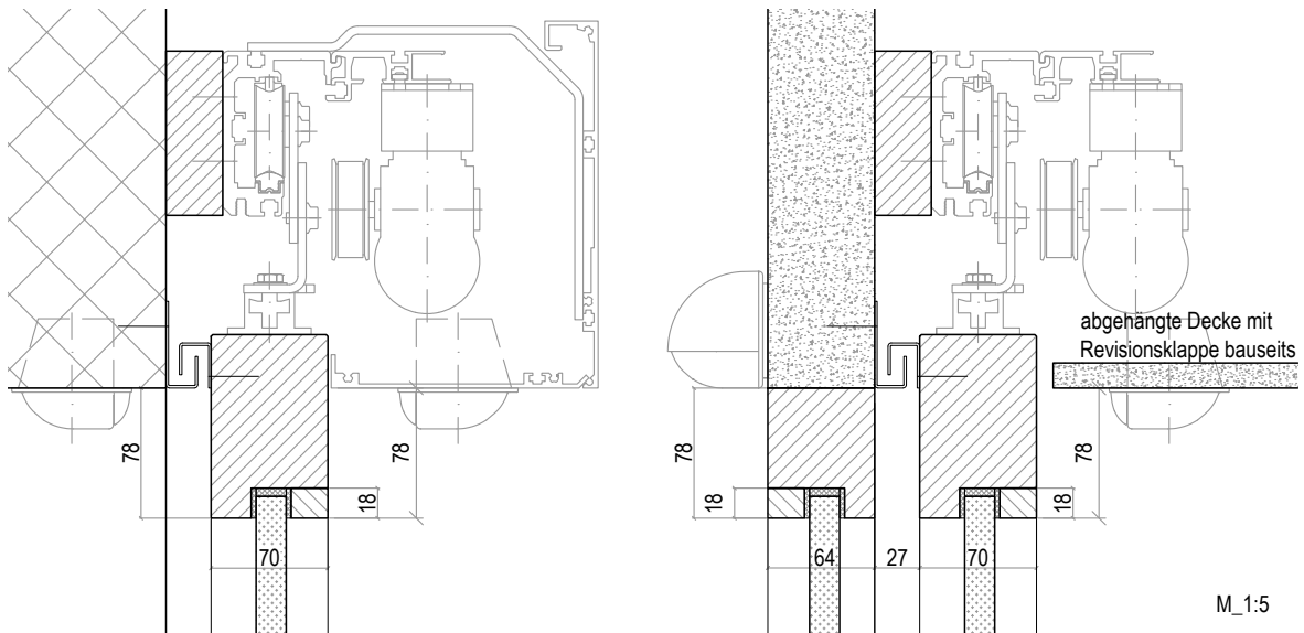
Sturzdetail (Vertikalschnitt)
