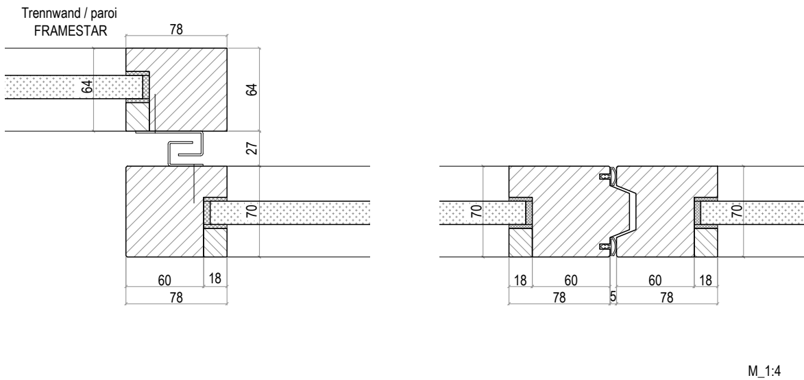
2-flüglige Ausführung, Anschluss Glaswand FRAMESTAR, Mitteldetail 2-flüglige Ausführung (Horizontalschnitt)
