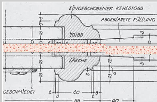
Detail Türblatt mit Einlage EI30 VKF
